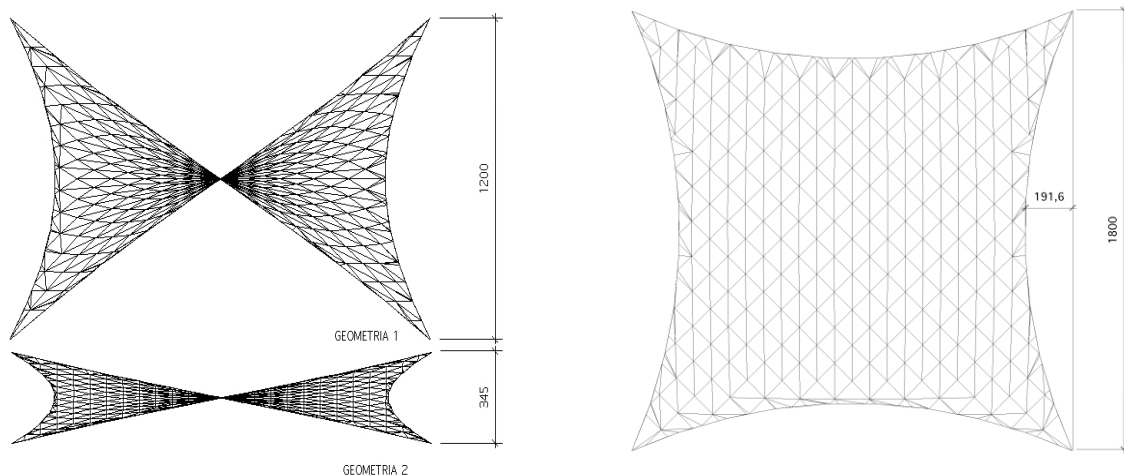
Figura.2 Geometría de los paraboloides de relaciones Flecha/luz 1:5(Geom.1), 1:15 (Geom.2).
