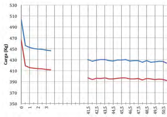
Grafico 3 Perdida de pretensión del Patrón.
