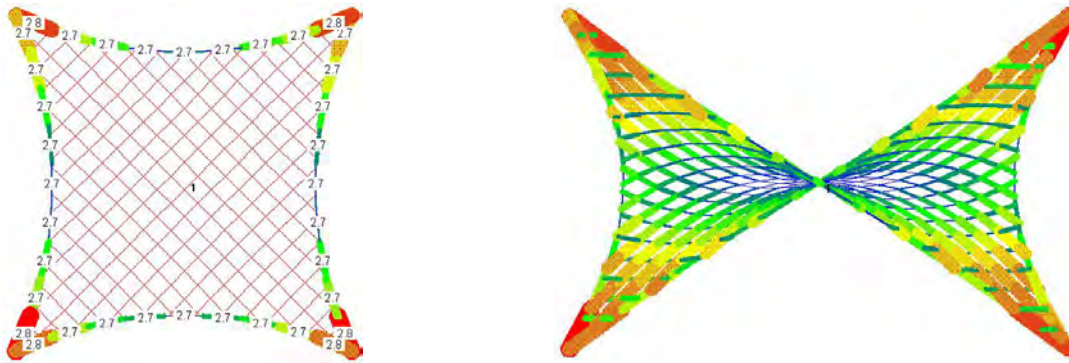
Figura.3 Salida grafica del programa donde se muestran las fuerzas resultantes en las relingas a la izquierda y sobre la superficie de la membrana a la derecha.
